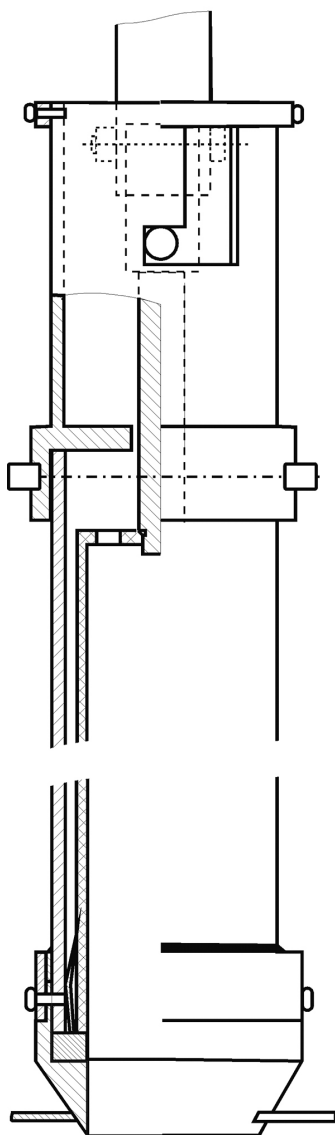
Рис. 2. Трубка-бур в разрезе.
